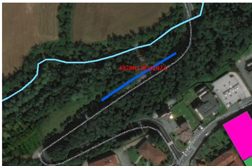
Figura 31 - Cedimento scarpata stradale per erosione del Torrente Serenza (in blu)
