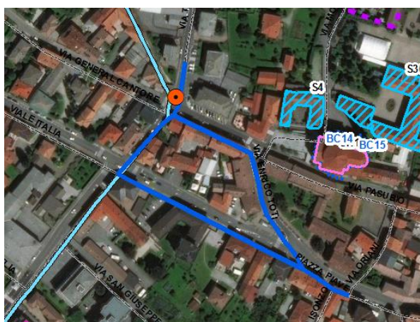
Figura 25 – Viabilità soggetta ad allagamento (in blu)
