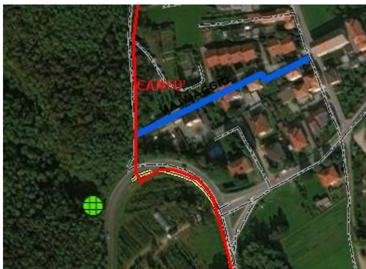
Figura 27 – Viabilità allagata in località Asnago (in blu) e scolmatore (in verde)
